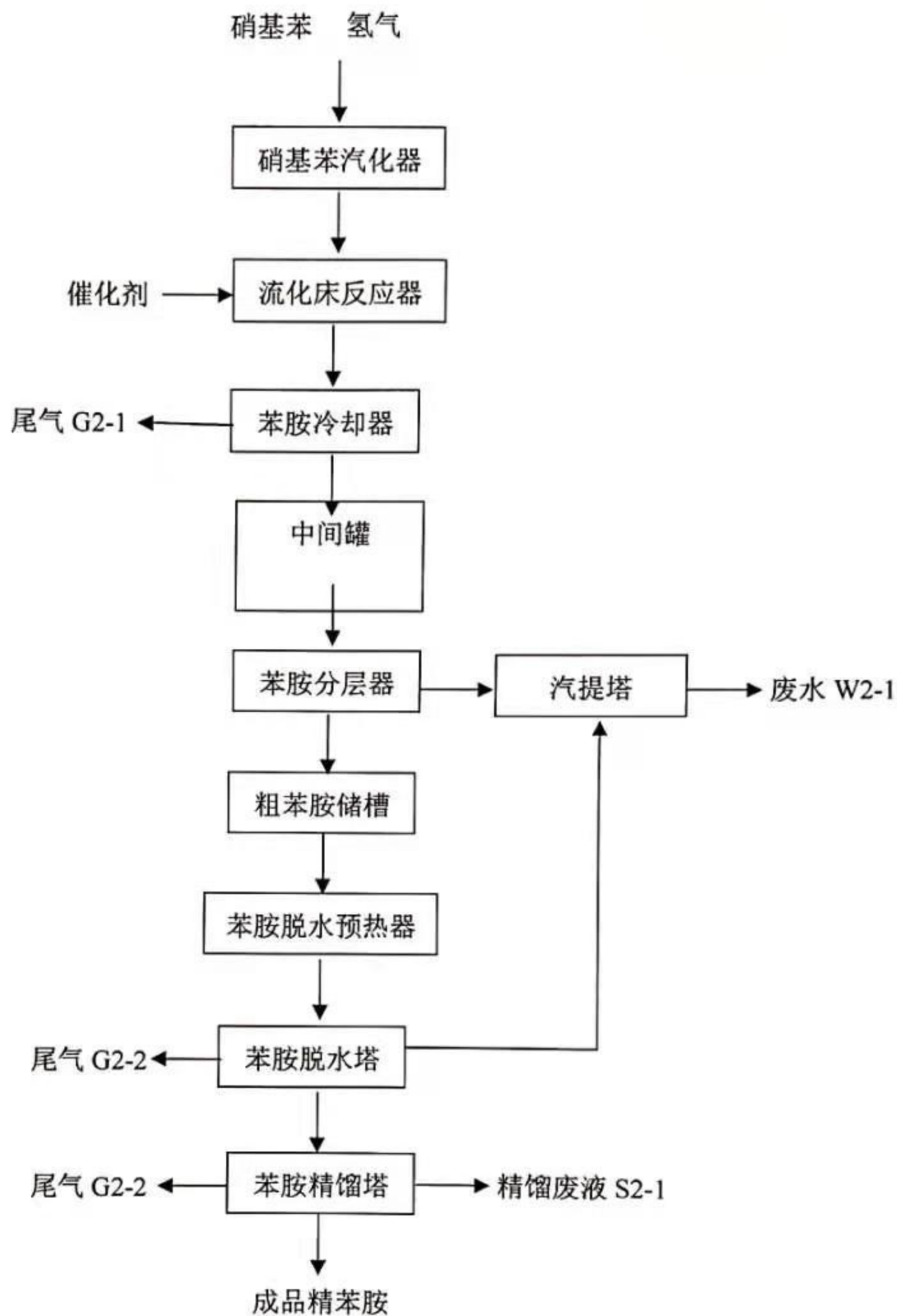
图 2.3-2 苯胺装置生产工艺流程及排污环节示意图
