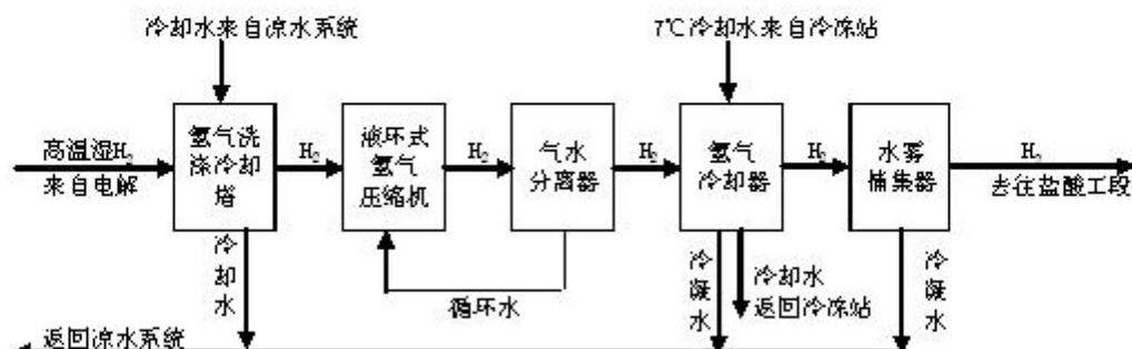
图 1-1-3 氢处理工段工艺流程及产物环节示意图-烧碱
