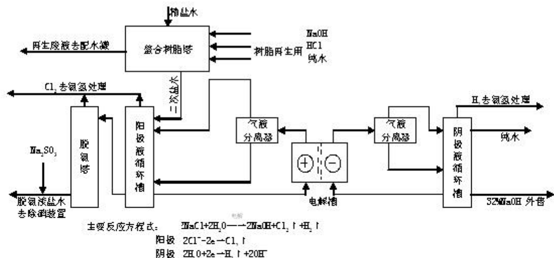
图 1-1-1 电解工段工艺流程及产物环节示意图-烧碱
