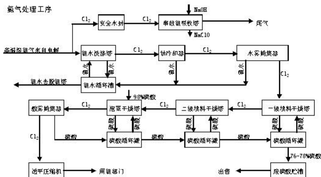
图 1-1-2 氯处理工段工艺流程及产物环节示意图-烧碱
